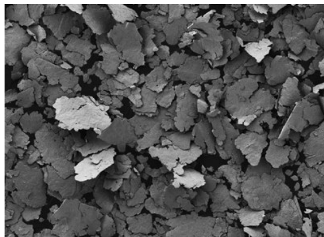
Repräsentative REM Aufnahme/ Representative SEM micrograph
