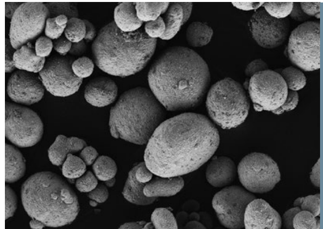
Repräsentative REM Aufnahme/ Representative SEM micrograph
